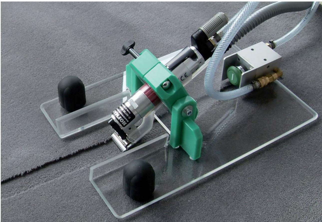
MS 40-A mit Grundplatte / MS 40-A with base plate
